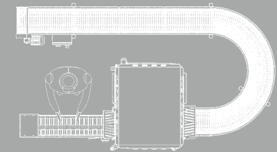
Beispiel für Aufstellung mit Kurvenförderer. Example for installation with curve conveyor.
